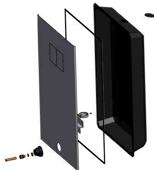
Läckageindikerande box, LI-Box.
